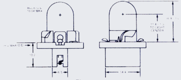
Fig. 120 T-3/4
