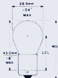
Fig. 29 S-8
