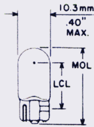
Fig. 77 T-3/4
