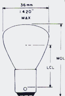
Fig. 25 RP-11
