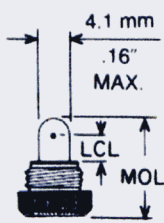
Fig. 40 T-1/4
