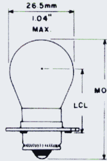
Fig. 31 S-8
