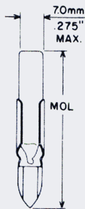
Fig. 58 T-2
