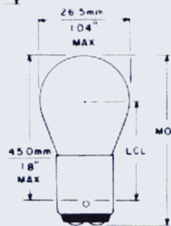
Fig. 30 S-8
