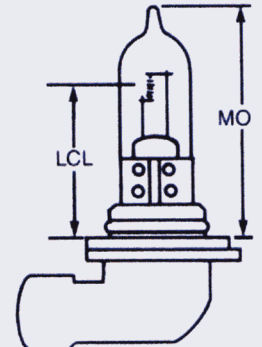
Fig. 122 T-3/4
