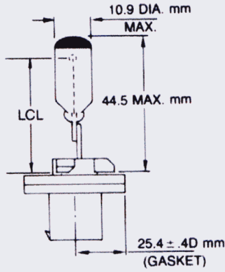
Fig. 115 T-3/4
