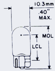
Fig. 77 T-3/4
