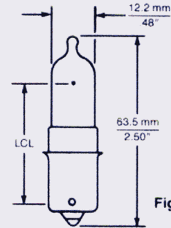
Fig. 123 T-3 1/2
