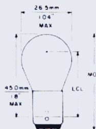
Fig. 33 S-8
