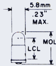
Fig. 50 T-1 3/4
