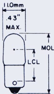
Fig. 76 T-3/4
