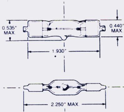
Fig. 107 T-3
