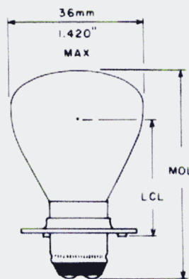
Fig. 27 RP-11
