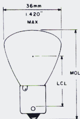
Fig. 26 RP-11
