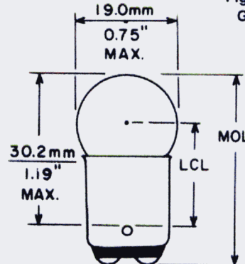
Fig. 17 G-6
