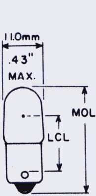
Fig. 76 T-3/4
