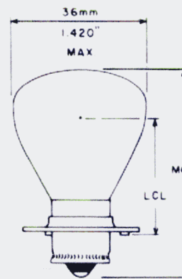
Fig. 27a RP-11
