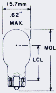
Fig. 86 T-5
