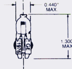
Fig. 110 T-3
