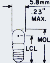
Fig. 51 T-1 1/4
