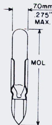
Fig. 61 T-2
