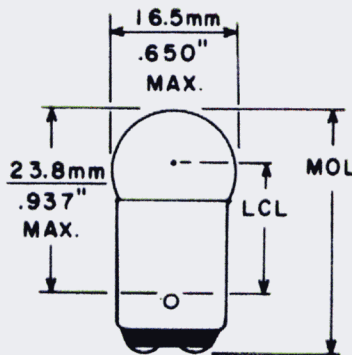
Fig. 13 G-5
