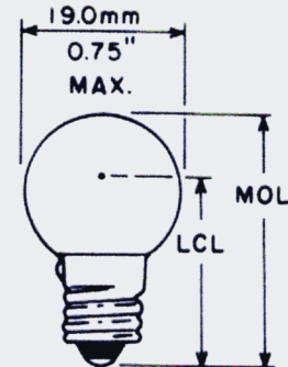
Fig. 15 G-6
