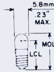
Fig. 51 T-1 3/4
