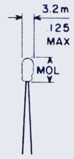
Fig. 37 T-1
