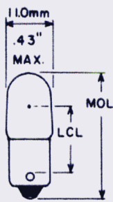
Fig. 76 T-3/4
