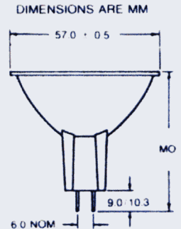
Fig. 104 PAR-18
