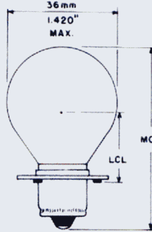
Fig. 34 S-11
