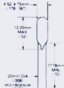
Fig. 96 T-1/2
