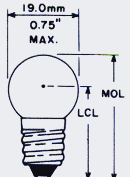
Fig. 18 G-6
