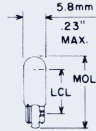
Fig. 52 T-1 3/4
