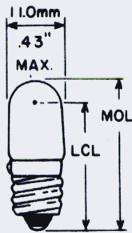
Fig. 75 T-3/4
