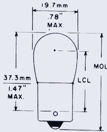
Fig. 2 B-6
